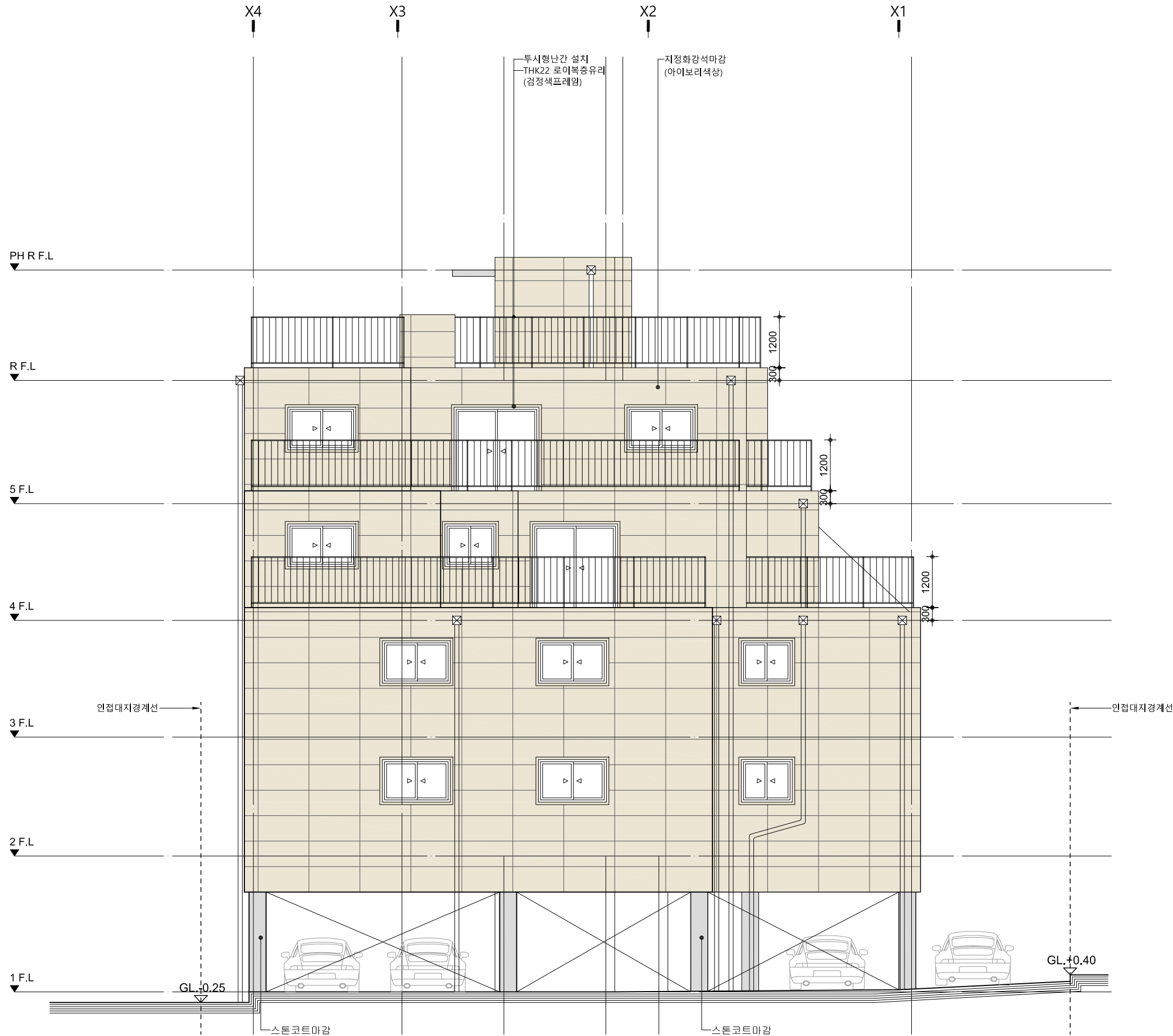
배면도(동측면도) SCALE A3 : 1/100
