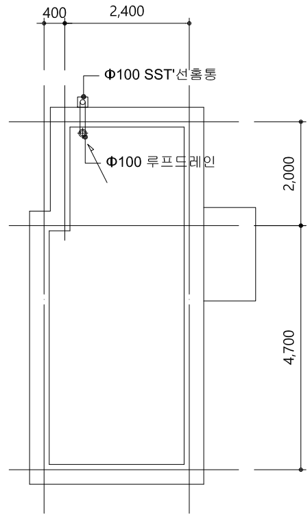
옥탑 지붕 평면도 SCALE A3 : 1/100
